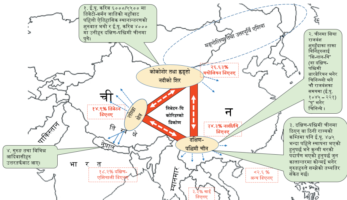
चित्र ८: तिबेटन-यि करिडरमा डिएनए तथा अन्य ऐतिहासिक तथ्यहरूको एकीकृत विश्लेषण
