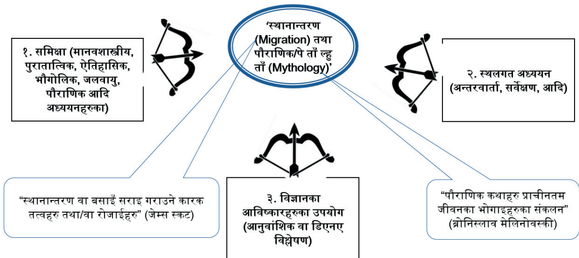
चित्र २: अध्ययनका लागि सैद्धान्तिक तथा विधिगत खाका
