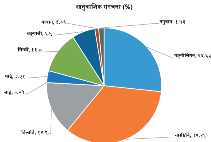
चित्र ५: पंक्तिकारको पैतृक आनुवांशिक संरचना
