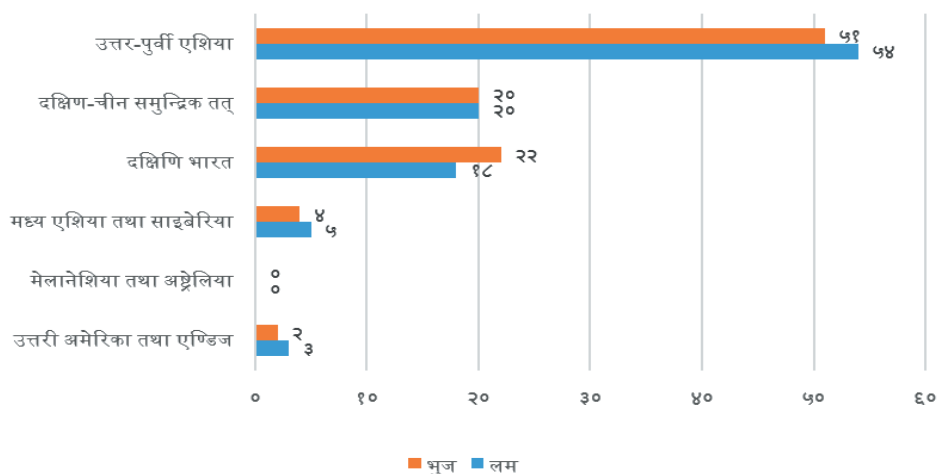
चित्र ७: भुज तथा लम गुरुङ व्यक्तिको आनुवांशिक संरचनाहरू
