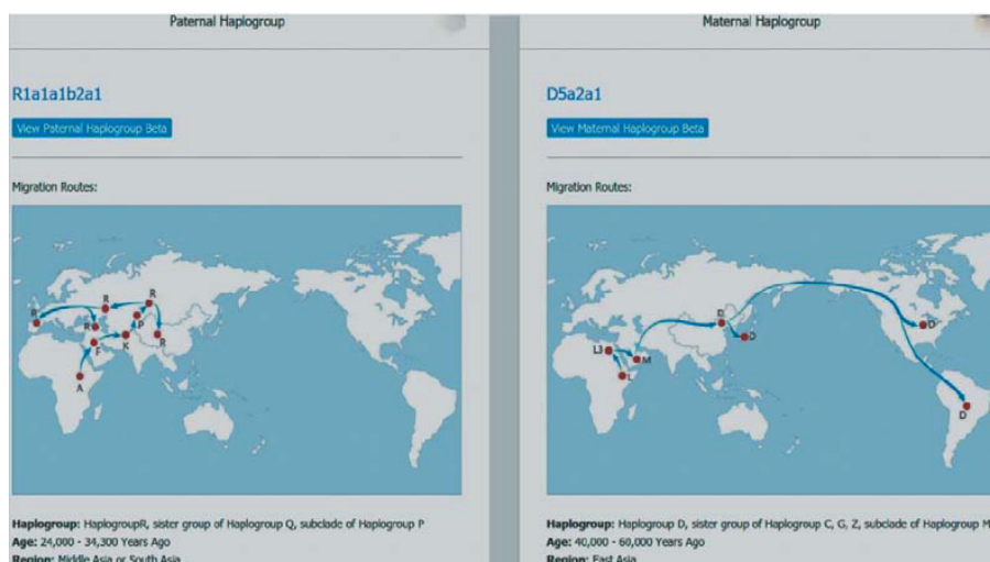
चित्र ६: बाबा तथा आमातर्फका प्राचीन पुर्खाहरू हिंडेका बाटाहरू
